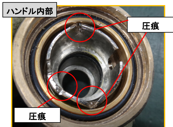
ハンドル内部(スライダー外観)
