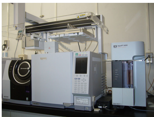
かび臭物質の測定に使用するガスクロマトグラフィー質量分析装置
